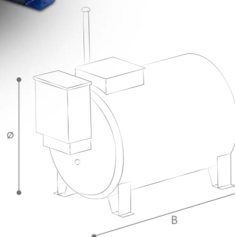
SERBATOIO MM.
